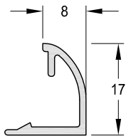
1020690 - Contravidrio Curvo 8 mm. Peso: 0,14 Kg/m. Largo Std.: 6.030 mm.
