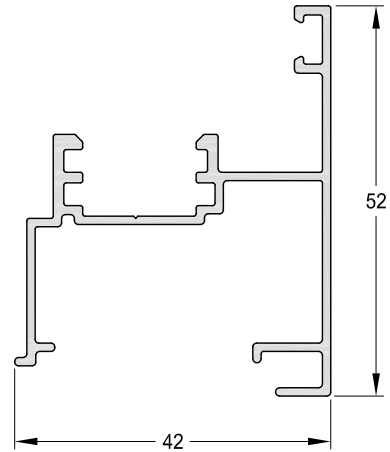
1032980 - Encuentro Central Ventana y Puerta de Rebatir Peso: 0,54 Kg/m. Largo Std.: 6.030 mm.
