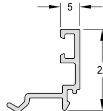
1020644 - Contravidrio Recto 5 mm. Peso: 0,18 Kg/m. Largo Std.: 6.030 mm.
