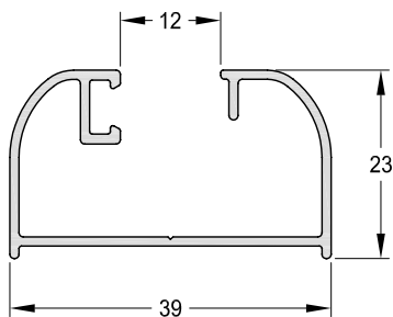
1032984 - Adaptador V.S. Peso: 0,35 Kg/m. Largo Std.: 6.030 mm.
