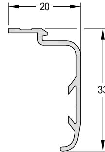
1010709 - Contramarco Peso: 0,19 Kg/m. Largo Std.: 6.150 mm.
