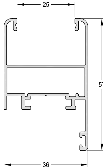
1032979 - Hoja D.V.H. Peso: 0,65 Kg/m. Largo Std.: 6.030 mm.
