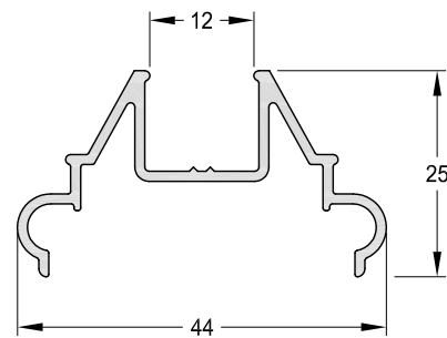
1011948 - Aplique Perimetral 12 mm. Peso: 0,35 Kg/m. Largo Std.: 6.030 mm.
