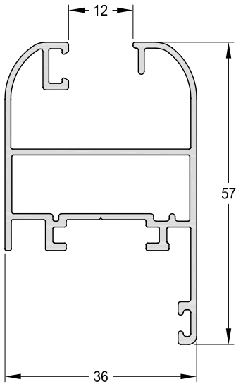
1032978 - Hoja V.S. Peso: 0,69 Kg/m. Largo Std.: 6.030 mm.
