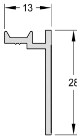
1010441 - Contramarco Peso: 0,18 Kg/m. Largo Std.: 6.150 mm.
