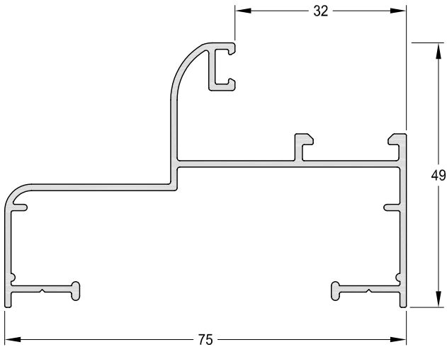
1032977 - Marco Peso: 0,72 Kg/m. Largo Std.: 6.200 mm.
