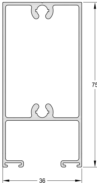
1032982 - Zócalo Peso: 1,01 Kg/m. Largo Std.: 6.030 mm.
