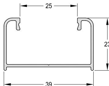
1032985 - Adaptador D.V.H. Peso: 0,30 Kg/m. Largo Std.: 6.030 mm.
