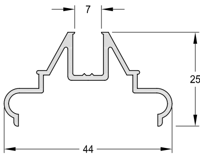
1011964 - Aplique Perimetral 7 mm. Peso: 0,35 Kg/m Largo Std.: 6.030 mm.
