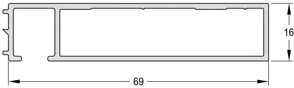
1050840 - Premarco Peso: 0,63 Kg/m. Largo Std.: 6.150 mm.
