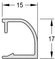
1020666 - Contravidrio Curvo 15 mm. Peso: 0,16 Kg/m. Largo Std.: 6.030 mm.
