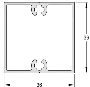
1032983 - Travesaño Peso: 0,61 Kg/m. Largo Std.: 6.030 mm.
