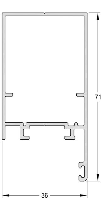
1032981 - Parante Peso: 0,79 Kg/m. Largo Std.: 6.200 mm.
