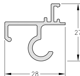
1060843 - Bisagra Tapacinta Peso: 0,34 Kg/m. Largo Std.: 6.150 mm.
