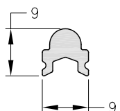
1060543 - Guía Inferior radio 3 mm Peso: 0,13 Kg/m Largo Std.: 6030 mm
