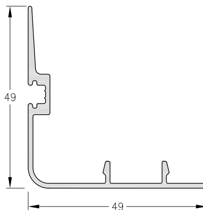
1060556 - Encuentro de hoja M-Cinco Peso: 0.46 Kg/m. Largo Std.: 6150 mm.
