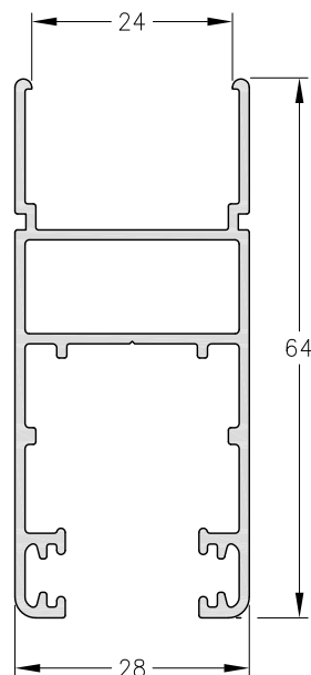
1060742 - Hoja Perimetral D.V.H. Peso: 0,72 Kg/m. Largo Std.: 6.030 mm.
