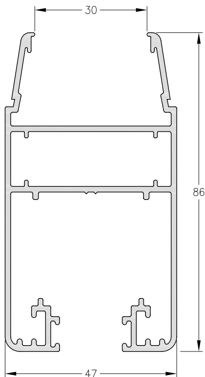
1060555 - Hoja Perimetral Peso: 1,43 Kg/m. Largo Std.: 6.150 mm.
