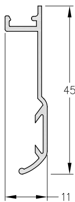
1060862 - Contramarca Peso: 0,21 Kg/m. Largo Std.: 6.150 mm.
