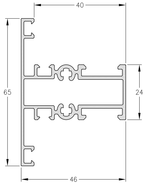
1060835 - Travesaño Angosto Peso: 0,94 Kg/m. Largo Std.: 6.030 mm.
