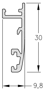
1060884 - Contramarca Peso: 0,20 Kg/m. Largo Std.: 6.150 mm.
