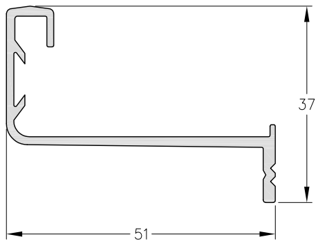
1060558 - Guía Mosquitero Peso: 0,49 Kg/m. Largo Std.: 6.030 mm.
