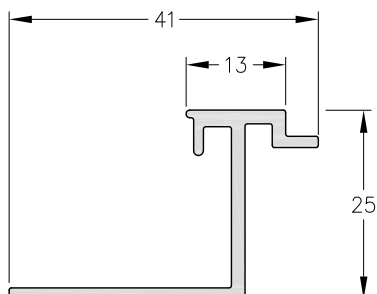
1060546 - Contravidro de 13,2 mm. Peso: 0,35 Kg/m. Largo Std.: 6.030 mm.
