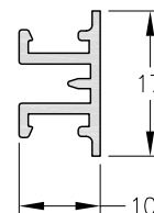
1060540 - Tapa Soporte Paño Fijo Peso: 0,15 Kg/m. Largo Std.: 6.030 mm.
