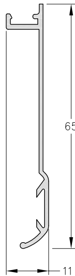
1060857 - Contramarca Peso: 0,27 Kg/m. Largo Std.: 6.150 mm.
