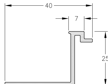
1060611 - Contravidro de 7,2 mm. Peso: 0,30 Kg/m. Largo Std.: 6.030 mm.
