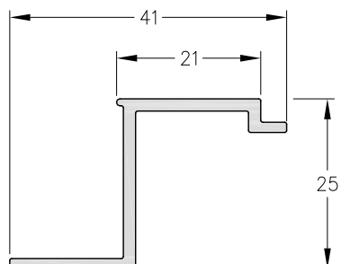
1060612 - Contravidro de 21,2 mm. Peso: 0,31 Kg/m. Largo Std.: 6.030 mm.
