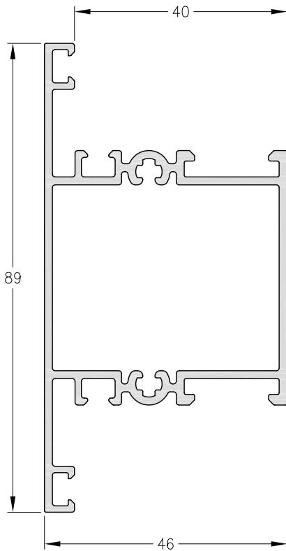
1060888 - Travesaño Ancho Peso: 1,21 Kg/m. Largo Std.: 6.030 mm.
