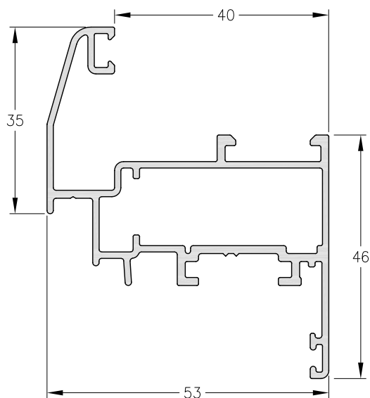
1060883 - Hoja V.R., B. y O.B. Peso: 0,90 Kg/m. Largo Std.: 6.150 mm.
