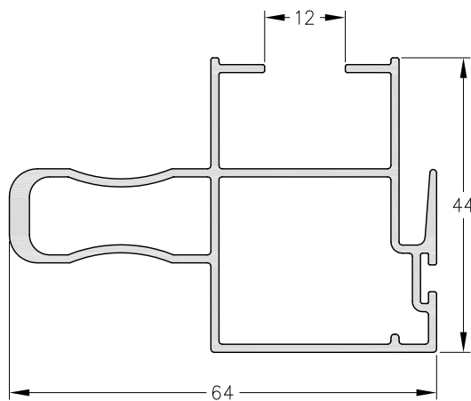
1060834 - Parante Central Ref. V.S. Peso: 0,88 Kg/m. Largo Std.: 6.150 mm.
