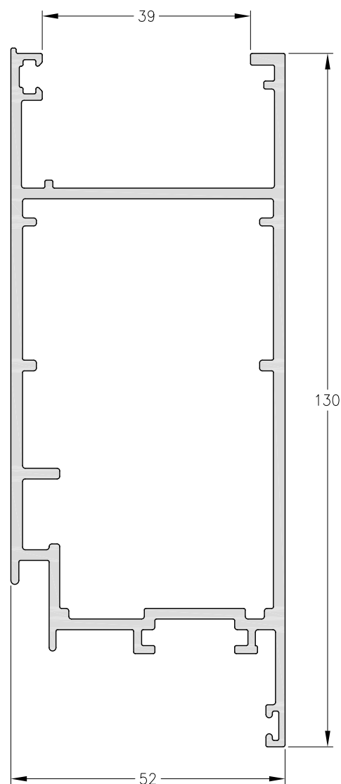
1060500 - Cabezal y Parante Reforzado Peso: 2,17 Kg/m. Largo Std.: 6.150 mm.
