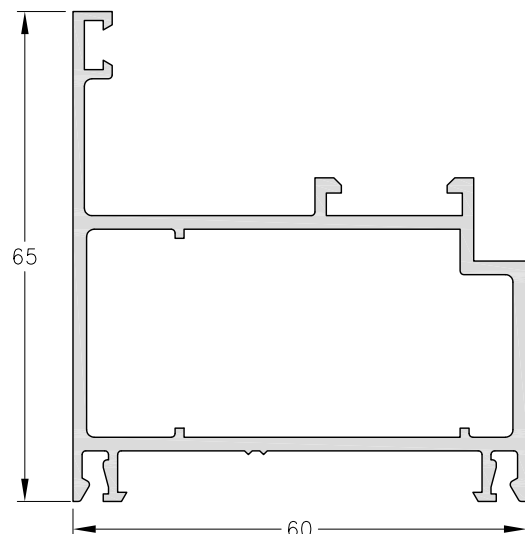
4040 - Marco Puerta Peso: 1,18 Kg/m. Largo Std.: 6.200 mm.
