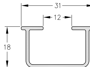
4000 - Adaptador VS en zócalo y dintel. Peso: 0.261 Kg/m. Largo Std.: 6.200 mm.
