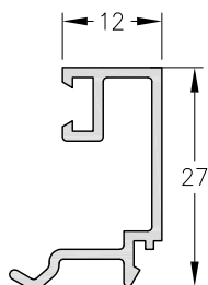
4049 - Contravidrio Recto L.E.. Peso: 0.232 Kg/m. Largo Std.: 6.200 mm.
