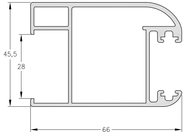
4071 - Parante lateral p/ DVH. Peso: 1.291Kg/m. Largo Std.: 6.200 mm. Largo Opc.: 4800 mm.
