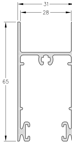
4073 - Zócalo y Cabezal p/ DVH. Peso: 0.861 Kg/m. Largo Std.: 6.200 mm.
