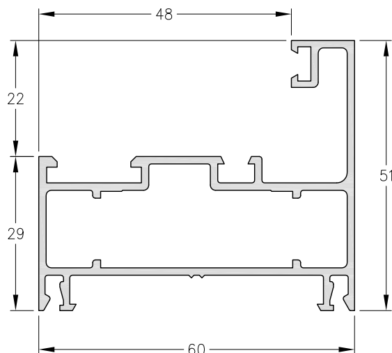
4059 - Marco Paño Fijo Recto, Ventana de Rebatir. Peso: 1.001 Kg/m. Largo Std.: 6.200 mm.
