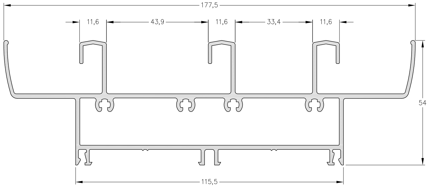
4081 - Umbral dintel de marco 3 guías.
