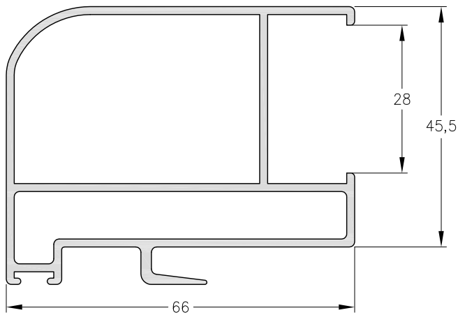
4082 - Parante ctral 3er hoja DVH. Peso: 1.267 Kg/m. Largo Std.: 6.200 mm.
