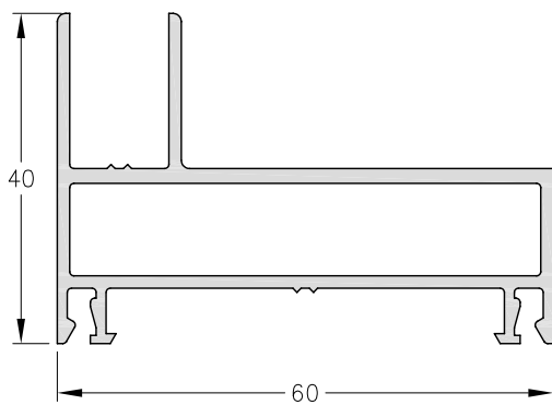
4036 - Jamba de marco.
