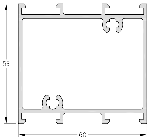
4042 - Travesaño Peso: 1,40 Kg/m. Largo Std.: 6.200 mm.
