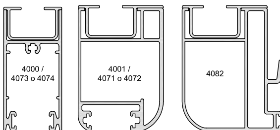
Detalle de montaje de adaptadores para Vidrio Simple ESC. 2:1
