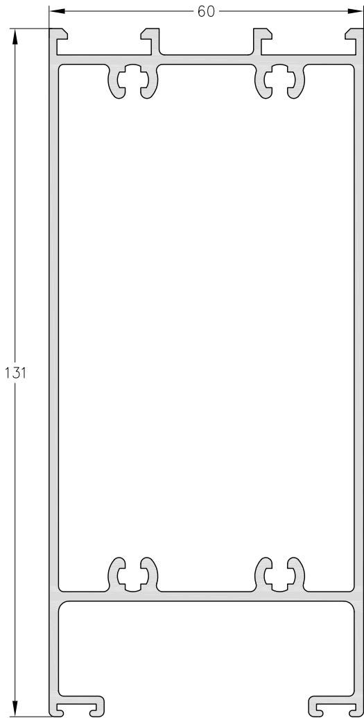
4043 - Zócalo Puerta Peso: 2,32 Kg/m. Largo Std.: 6.200 mm.
