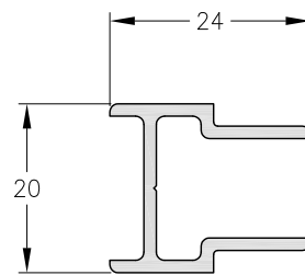
4965 - Encuentro central Corrediza 4 Hojas Peso: 0,29 Kg/m. Largo Std.: 6.200 mm.
