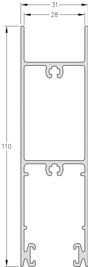
4074 - Zócalo alto p/ DVH. Peso: 1.407 Kg/m. Largo Std.: 6.200 mm.
