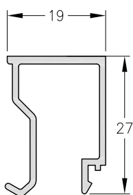
4046 - Contravidrio Recto P/DVH. Peso: 0.273 Kg/m. Largo Std.: 6.200 mm.
