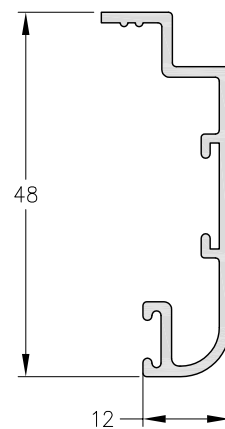
3083 - Contramarco p/ Atornillar.
