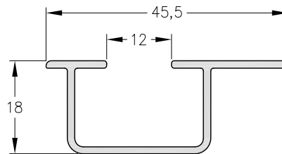
4001 - Adaptador VS en parantes. Peso: 0.324 Kg/m. Largo Std.: 6.200 mm.
