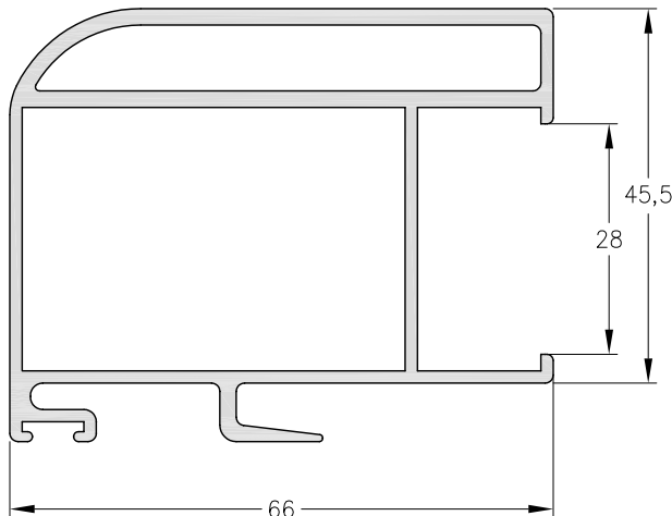
4072 - Parante central p/ DVH. Peso: 1.466 Kg/m. Largo Std.: 6.200 mm. Largo Opc.: 4800 mm.
