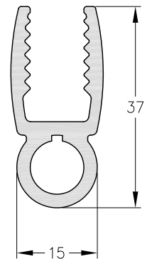
1090203 - Hoja Peso: 0,64 Kg/m. Largo Std.: 6.030 mm.
