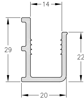
1090031 - Porta Blisan Inferior Peso: 0,38 Kg/m. Largo Std.: 6.030 mm.
