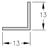
1090751 - Perfil Angulo Peso: 0,08 Kg/m. Largo Std.: 6.030 mm.
