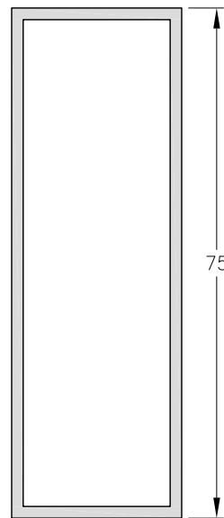
1090457 - Tubo 75 x 25 mm. Peso: 0,90 Kg/m. Largo Std.: 6.030 mm.
