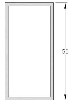
1090809 - Tubo 50 x 25 mm. Peso: 0,55 Kg/m. Largo Std.: 6.030 mm.
