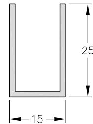
1090650 - "U" de Blindex Peso: 0,25 Kg/m. Largo Std.: 6.030 mm.
