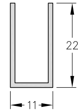
1090466 - "U" 11,1 x 22 mm Peso: 0,17 Kg/m. Largo Std.: 6.030 mm.
