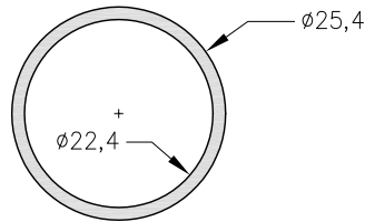
1090995 - Caño Redondo Peso: 0,31 Kg/m. Largo Std.: 6.030 mm.
