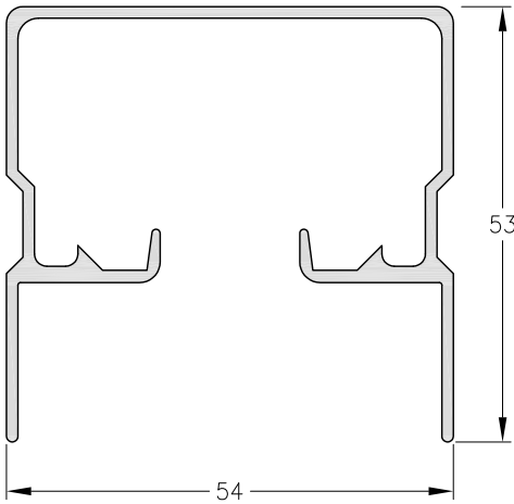
1090941 - Cabezal Peso: 0,82 Kg/m. Largo Std.: 6.030 mm.
