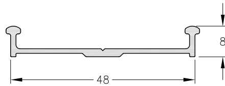
1090157 - Guía Inferior Peso: 0,25 Kg/m. Largo Std.: 6.030 mm.
