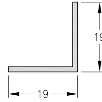
1090753 - Perfil Angulo Peso: 0,14 Kg/m. Largo Std.: 6.030 mm.
