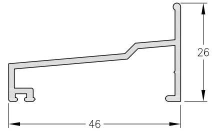
1090942 - Umbral Peso: 0,37 Kg/m. Largo Std.: 6.030 mm.
