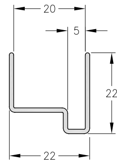
1090158 - Cantonera de 18 mm. Peso: 0,20 Kg/m. Largo Std.: 6.030 mm.
