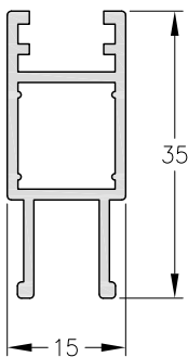
1090944 - Hoja Peso: 0,35 Kg/m. Largo Std.: 6.030 mm.
