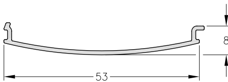
1090029 - Tapa Inferior Pasamanos Curvo Peso: 0,20 Kg/m. Largo Std.: 6.030 mm.
