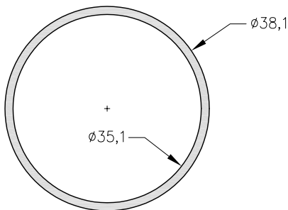
1090996 - Caño Redondo Peso: 0,47 Kg/m. Largo Std.: 6.030 mm.
