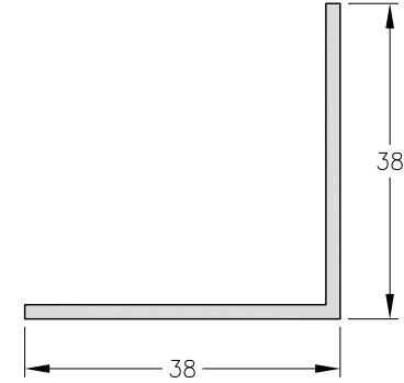
1090757 - Perfil Angulo Peso: 0,34 Kg/m. Largo Std.: 6.030 mm.
