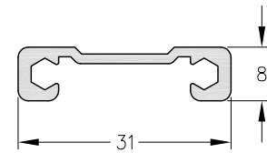
1090946 - Barra Toallera Peso: 0,24 Kg/m. Largo Std.: 6.030 mm.
