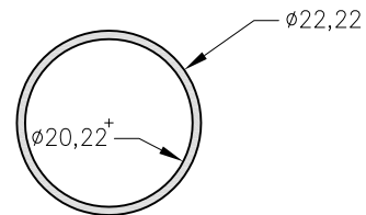
3085 - Caño Redondo Peso: 0,18 Kg/m. Largo Std.: 6.030 mm.
