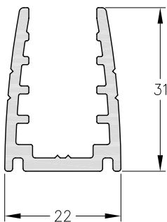
1090201 - Marco Peso: 0,52 Kg/m. Largo Std.: 6.030 mm.
