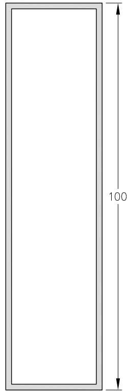
1090461 - Tubo 100 x 25 mm. Peso: 0,99 Kg/m. Largo Std.: 6.030 mm.
