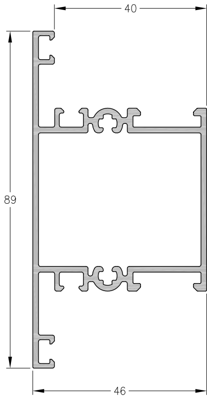
1060888 - Travesañó Ancho Peso: 1,21 Kg/m. Largo Std.: 6.030 mm.
