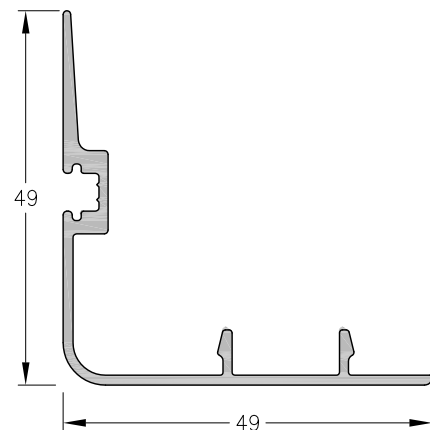
1060556 - Encuentro de hoja M-Cinco Peso: 0.46 Kg/m. Largo Std.: 6150 mm.
