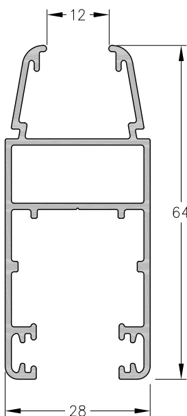
1060787 - Hoja Perimetral V. Laminado Peso: 0,76 Kg/m. Largo Std.: 6.030 mm.
