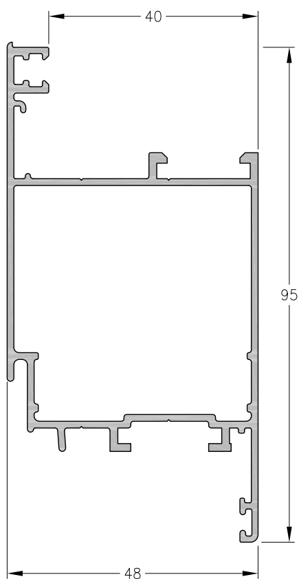
1060861 - Cabezal y Parante Peso: 1,10 Kg/m. Largo Std.: 6.150 mm.
