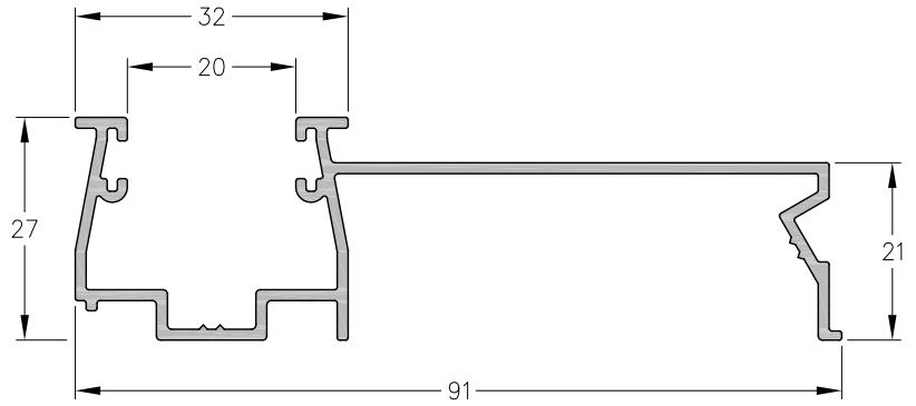
153 - Guía de Cortina Común Peso: 0,70 Kg/m Largo Std.: 6150 mm
