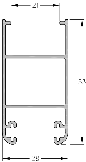
1060819 - Parante Lateral D.V.H. Peso: 0,61 Kg/m. Largo Std.: 6.150 mm.
