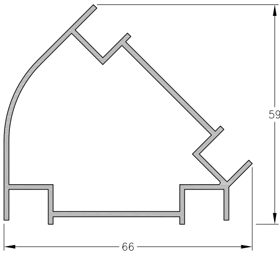
1060563 - Columna Curva a 135° Peso: 0,85 Kg/m. Largo Std.: 6.030 mm.
