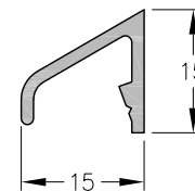
1060200 - Bota-Agua Peso: 0,15 Kg/m. Largo Std.: 6.030 mm.
