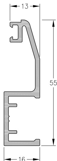
1060859 - Soporte Vidrio Paño Fijo Peso: 0,57 Kg/m. Largo Std.: 6.030 mm.
