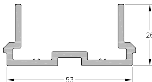
1060600 - Base Inercial Peso: 0,80 Kg/m. Largo Std.: 6.030 mm.
