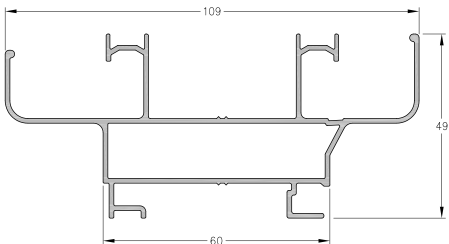
1060697 - Marco Perimetral Peso: 1,20 Kg/m. Largo Std.: 6.150 mm.
