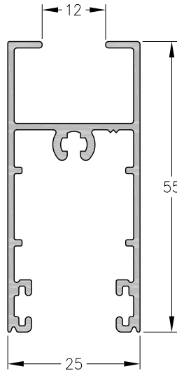
1060820 - Cabezal / Zócalo V.S. Peso: 0,62 Kg/m. Largo Std.: 6.030 mm.
