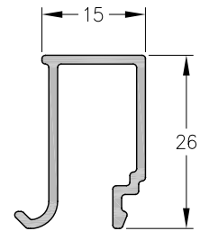
1060878 - Contravidrio Peso: 0,25 Kg/m. Largo Std.: 6.030 mm.
