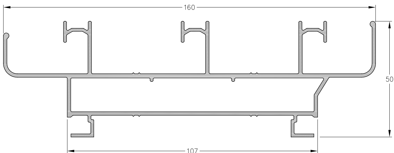
1060873 - Marco Perimetral de Tres Guías Peso: 2,10 Kg/m. Largo Std.: 6.150 mm.
