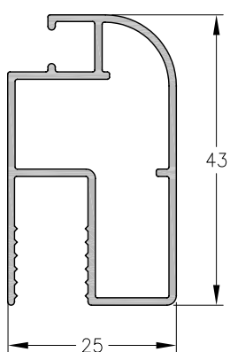
1060108 - Hoja Mosquitero Peso: 0,47 Kg/m. Largo Std.: 6.030 mm.
