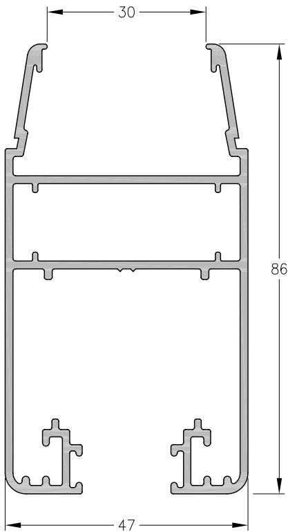
1060555 - Hoja Perimetral Peso: 1,43 Kg/m. Largo Std.: 6.150 mm.
