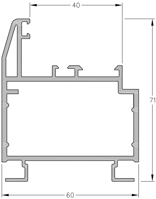
1060541 - Marco Peso: 1,57 Kg/m. Largo Std.: 6.150 mm.
