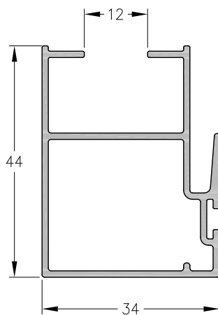
1060822 - Parante Central V.S. Peso: 0,60 Kg/m. Largo Std.: 6.150 mm.
