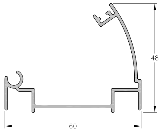
1060595 - Rótula Interior Peso: 0,58 Kg/m. Largo Std.: 6.030 mm.
