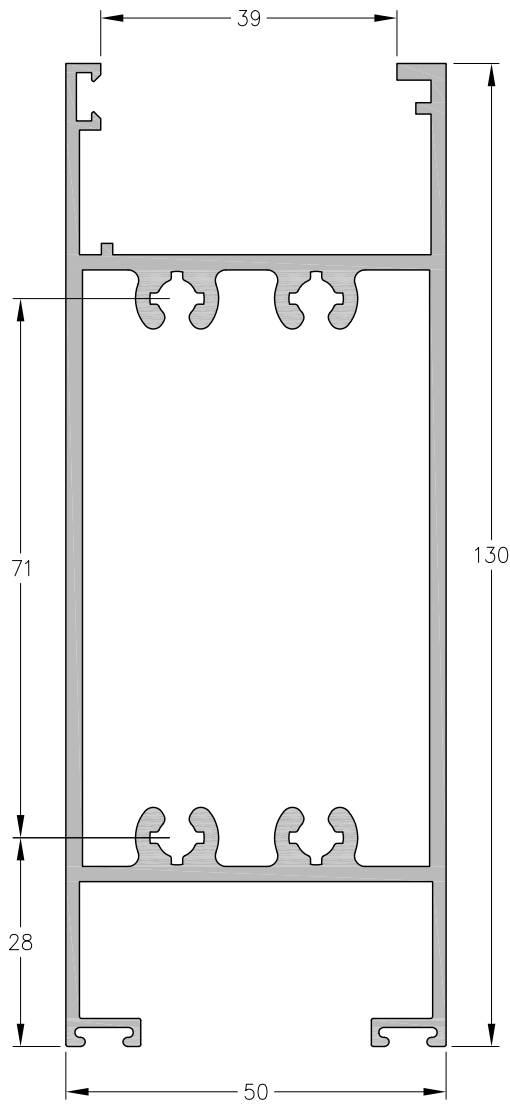
1060542 - Zócalo Reforzado Peso: 2,55 Kg/m. Largo Std.: 6.030 mm.
