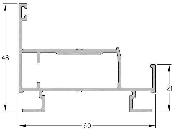
1060785 - Marco Ventana Desplazable Peso: 0,82 Kg/m. Largo Std.: 6.030 mm.
