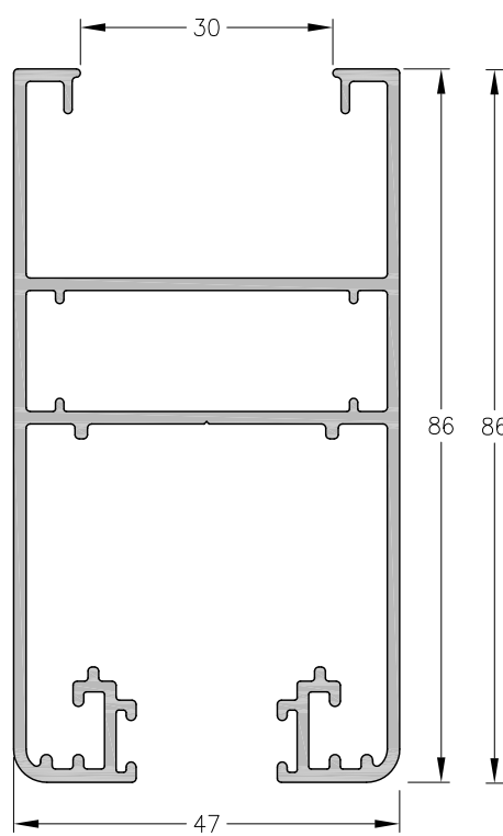
1060589 - Hoja recta DVH M-Cinco Peso: 1.43 Kg/m. Largo Std.: 6150 mm.
