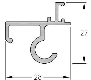
1060843 - Bisagra Tapacinta Peso: 0,34 Kg/m. Largo Std.: 6.150 mm.
