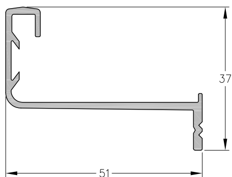
1060558 - Guía Mosquitero Peso: 0,49 Kg/m. Largo Std.: 6.030 mm.
