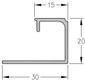
1060559 - Contravidrio 16 mm. para Perfil 1060555 Peso: 0,24 Kg/m. Largo Std.: 6.030 mm.
