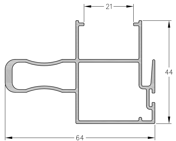
1060817 - Parante Central Ref. D.V.H. Peso: 0,85 Kg/m. Largo Std.: 6.150 mm.
