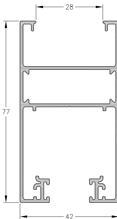
1060853 - Hoja Corrediza M-Tres recta DVH Peso: 1,15 Kg/m Largo Std.: 6150 mm
