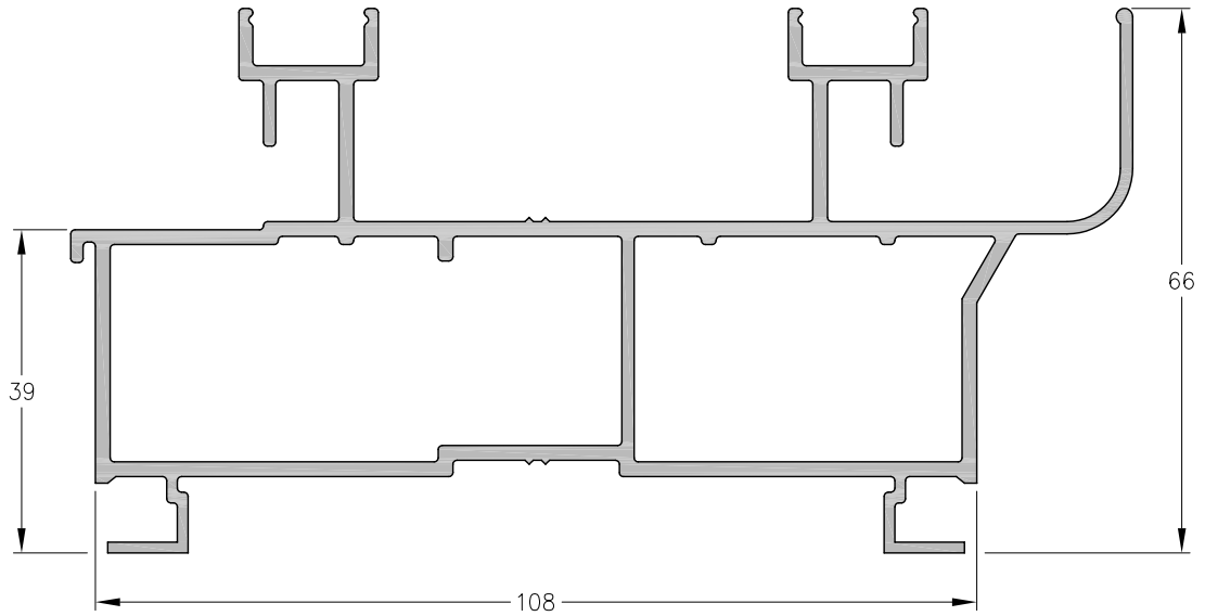
1060601 - Marco Peso: 2,35 Kg/m. Largo Std.: 6.150 mm.
