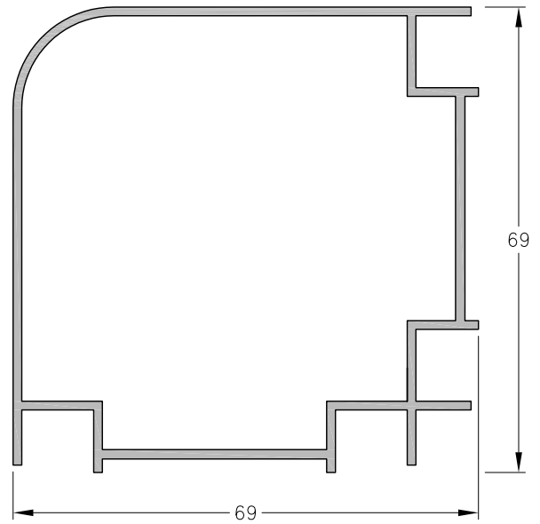
1060564 - Columna Curva a 90° Peso: 1,07 Kg/m. Largo Std.: 6.030 mm.
