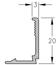
1060699 - Contravidrio Peso: 0,13 Kg/m. Largo Std.: 6.030 mm.
