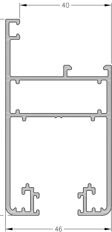
1060580 - Hoja Perimetral con Contravidrio Peso: 1,54 Kg/m. Largo Std.: 6.150 mm.
