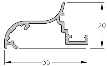
1060727 - Embellecedor de Marco Peso: 0,26 Kg/m. Largo Std.: 6.030 mm.
