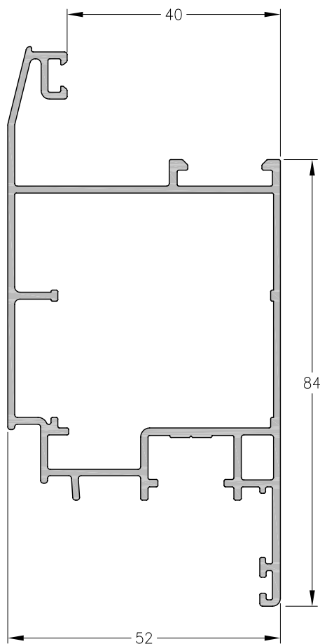
1060889 - Hoja C-16 Peso: 1,30 Kg/m. Largo Std.: 6.150 mm.
