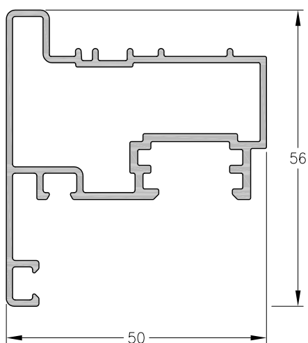
1060825 - Inversor Peso: 0,84 Kg/m. Largo Std.: 6.150 mm.
