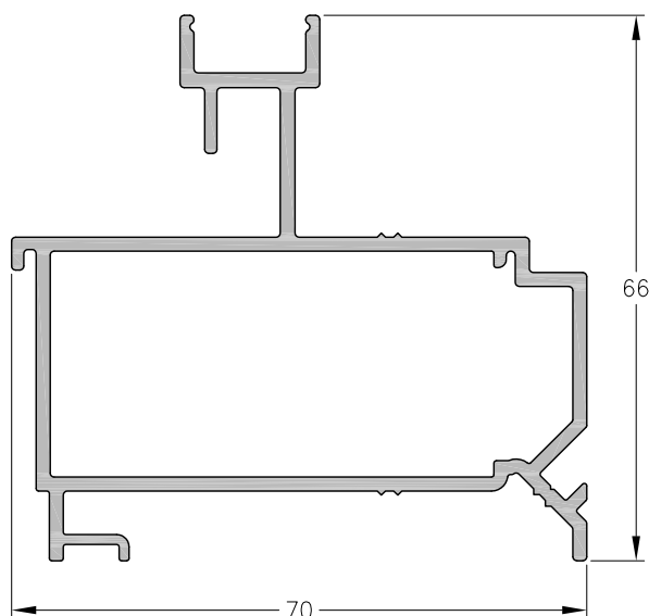
1060603 - Marco postizo Peso: 1,30 Kg/m Largo Std.: 6150 mm
