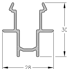
1060569 - Encuentro Cuatro Hojas M-Tres y M-Cinco Peso: 0,33 Kg/m. Largo Std.: 6.030 mm.
