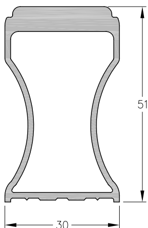
1060518 - Refuerzo Parantes M-Uno, M-Tres y M-Cinco Peso: 1,00 Kg/m. Largo Std.: 6.030 mm.
