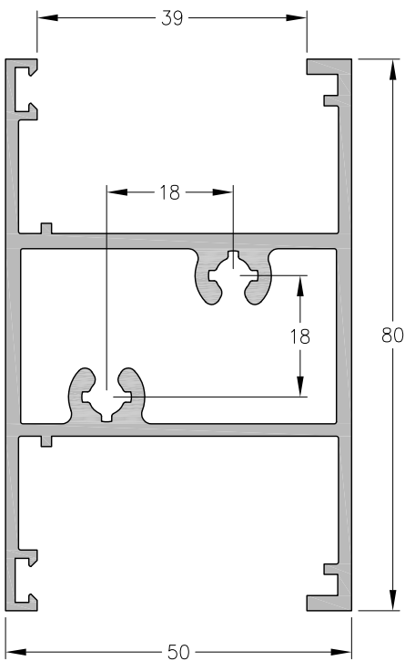
1060544 - Travesaño Peso: 1,71 Kg/m. Largo Std.: 6.030 mm.
