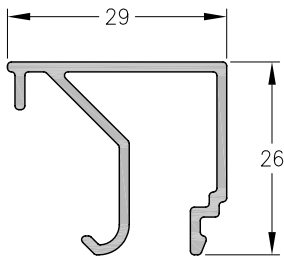
1060876 - Contravidrio Peso: 0,33 Kg/m. Largo Std.: 6.030 mm.
