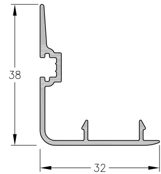
1060743 - Encuentro de hoja M-Uno Peso: 0.31 Kg/m. Largo Std.: 6.030 mm.
