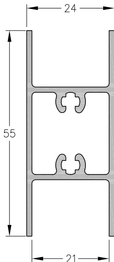
1020681 - Travesaño para hoja N-Uno Peso: 0,70 Kg/m. Largo Std.: 6.030 mm.
