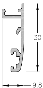
1060884 - Contramarca Peso: 0,20 Kg/m. Largo Std.: 6.150 mm.
