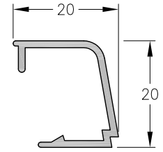
1060525 - Contravidrio Peso: 0,19 Kg/m. Largo Std.: 6.030 mm.
