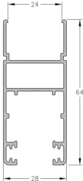
1060742 - Hoja Perimetral D.V.H. Peso: 0,72 Kg/m. Largo Std.: 6.030 mm.
