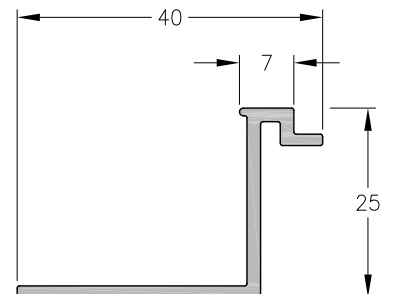
1060611 - Contravidrio de 7,2 mm. Peso: 0,30 Kg/m. Largo Std.: 6.030 mm.
