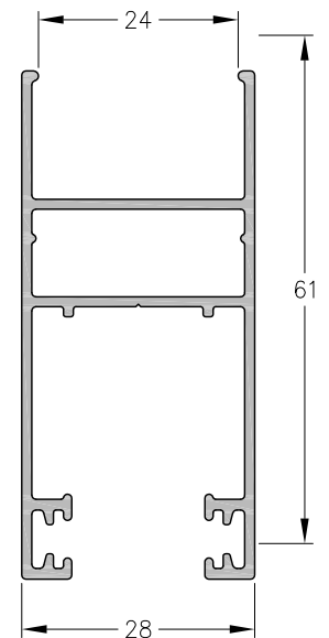
1060406 - Hoja corrediza DVH Peso: 0,68 Kg/m Largo Std.: 6030 mm
