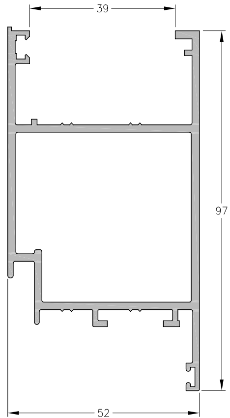
1060547 - Cabezal y Parante de Hoja Peso: 1,66 Kg/m. Largo Std.: 6.150 mm.
