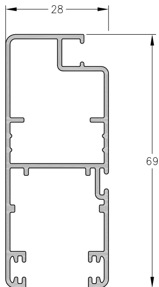
1060738 - Mosquitero Reforzado peso: 0,80 Kg/m
