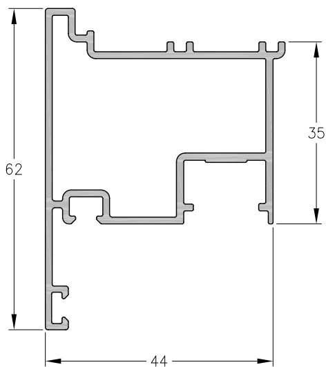
1060892 - Inversor C-16 Peso: 0,82 Kg/m. Largo Std.: 6.150 mm.
