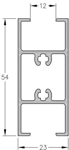
1020638 - Travesaño para hoja N-Uno Peso: 0,73 Kg/m Largo Std.: 6030 mm
