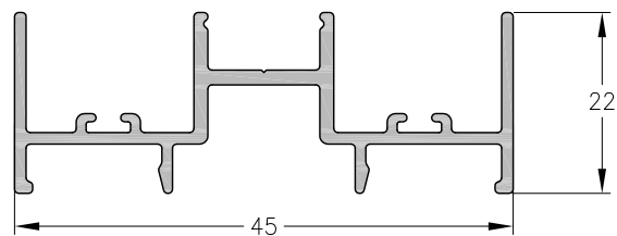
1060607 - Encuentro de Cuatro Hojas Peso: 0,62 Kg/m. Largo Std.: 6.030 mm.
