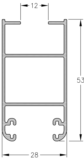
1060823 - Parante Lateral V.S. Peso: 0,64 Kg/m. Largo Std.: 6.150 mm.
