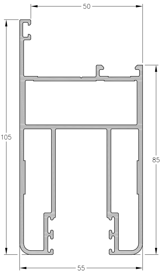
1060602 - Hoja Peso: 2,33 Kg/m. Largo Std.: 6.150 mm.
