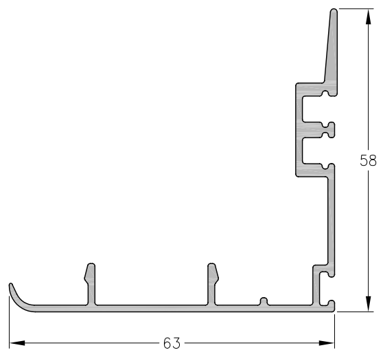
1060609 - Encuentro Peso: 0,66 Kg/m. Largo Std.: 6.150 mm.
