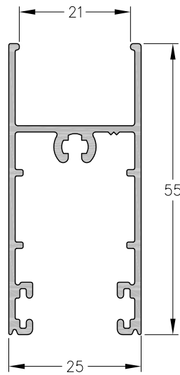
1060815 - Cabezal / Zócalo D.V.H. Peso: 0,59 Kg/m. Largo Std.: 6.030 mm.
