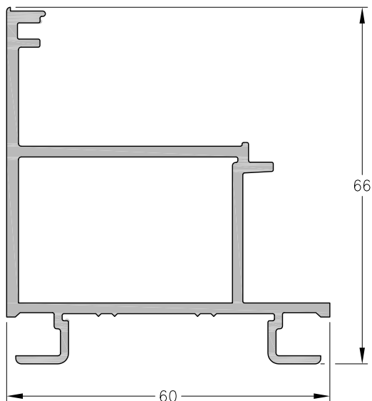
1060860 - Marco Paño Fijo Peso: 1,19 Kg/m. Largo Std.: 6.030 mm.
