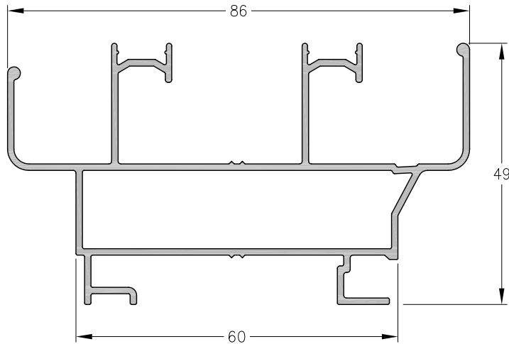
1060802 - Marco Perimetral Peso: 1,09 Kg/m. Largo Std.: 6.030 mm.
