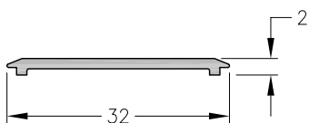
1060565 - Tapa Puerta Vaivén Peso: 0,13 Kg/m. Largo Std.: 6.030 mm.
