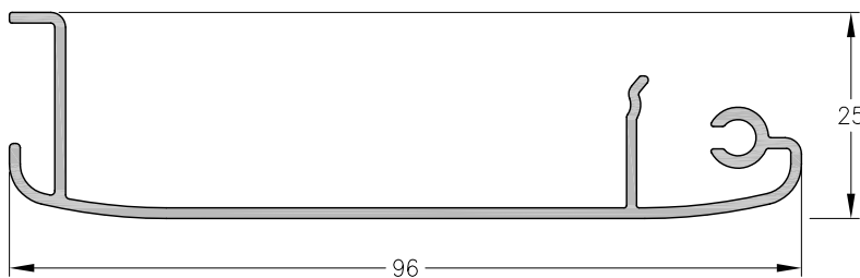
1060683 - Tapacinta Peso: 0,60 Kg/m. Largo Std.: 6.150 mm.
