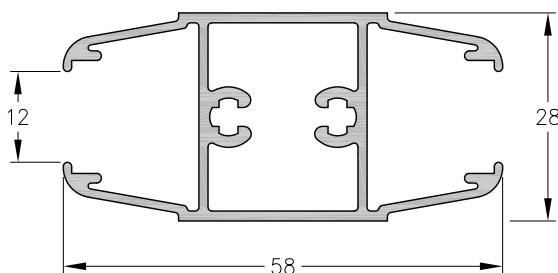
1060730 - Travesaño Hoja 1060787 Peso: 0,80 Kg/m. Largo Std.: 6.030 mm.
