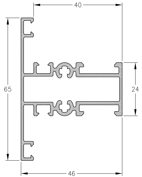
1060835 - Travesañó Angosto Peso: 0,94 Kg/m. Largo Std.: 6.030 mm.
