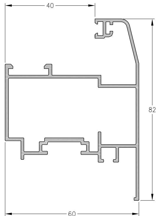
1060786 - Hoja Ventana Desplazable Peso: 1,18 Kg/m. Largo Std.: 6.030 mm.
