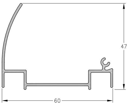
1060596 - Rótula Exterior Peso: 0,50 Kg/m. Largo Std.: 6.030 mm.
