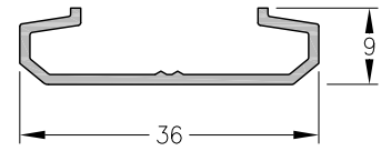
1060562 - Perfil de Fijación Inferior Marco-Premarco Peso: 0,19 Kg/m. Largo Std.: 6.030 mm.
