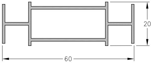
1060568 - Acople Recto Peso: 0,56 Kg/m. Largo Std.: 6.030 mm.
