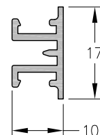
1060540 - Tapa Soporte Paño Fijo Peso: 0,15 Kg/m. Largo Std.: 6.030 mm.
