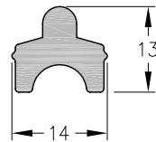
1060608 - Sobre Guía Marco Peso: 0,26 Kg/m. Largo Std.: 6.030 mm.
