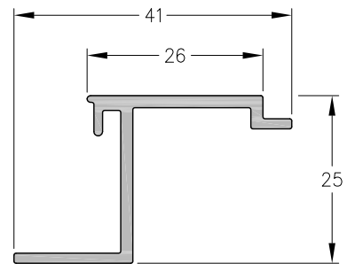
1060545 - Contravidrio de 26 mm. Peso: 0,35 Kg/m. Largo Std.: 6.030 mm.
