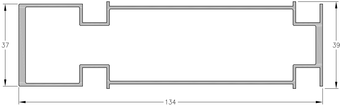
1060854 - Acople Recto Reforzado Peso: 1,60 Kg/m. Largo Std.: 6.030 mm.
