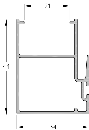
1060816 - Parante Central D.V.H. Peso: 0,57 Kg/m. Largo Std.: 6.150 mm.
