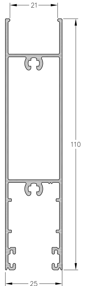
1060818 - Zócalo Alto D.V.H. Peso: 1,08 Kg/m. Largo Std.: 6.030 mm.
