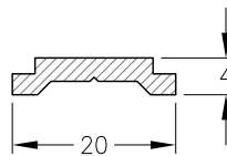
9469 - Pletina de Poliamida Largo Std.: 6.150 mm.
