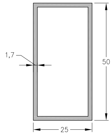
1090809 - Tubo 50 x 25 mm. Peso: 0,55 Kg/m. Largo Std.: 6.030 mm.
