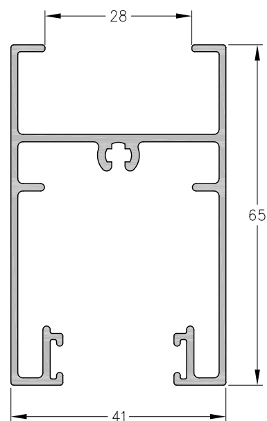
1110724 - Zócalo /cabezal hoja 90° DVH 28 mm Largo Std.: 6030 mm peso: 0,91 Kg/m
