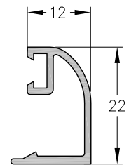
4050 - Contravidrio Curvo L.E.. Peso: 0.191 Kg/m. Largo Std.: 6.200 mm.
