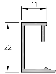
1110053 - Contravidrio recto 11 mm para clip Largo Std.: 6030 mm peso: 0,19 Kg/m
