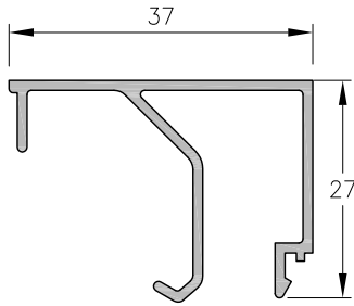
4045 - Contravidrio Recto 37 mm. Peso: 0.351 Kg/m. Largo Std.: 6.200 mm.
