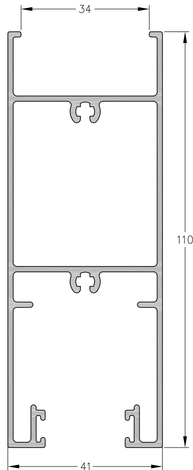
1110869 - Zócalo alto hoja corte 90° DVH Peso: 1,47 Kg/m Largo Std.: 6030 mm
