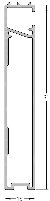
1060875 - Premarco largo std.: 6150 mm peso: 0,88 Kg/m
