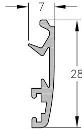
1020657 - Contramarco Peso: 0,19 Kg/m Largo Std.: 6150 mm
