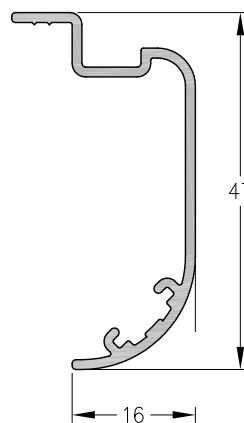
1020641 - Contramarco Peso: 0,32 Kg/m Largo Std.: 6150 mm
