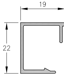
1110052 - Contravidrio recto 19 mm para clip Largo Std.: 6030 mm peso: 0,21 Kg/m
