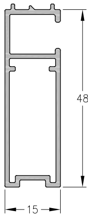
1060647 - Premarco de 48 mm. Peso: 0,46 Kg/m. Largo Std.: 6.150 mm.
