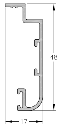
3083 - Contramarco Peso: 0,35 Kg/m Largo Std.: 6150 mm
