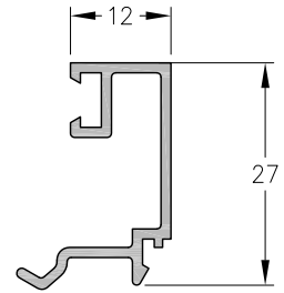
4049 - Contravidrio Recto L.E.. Peso: 0.232 Kg/m. Largo Std.: 6.200 mm.
