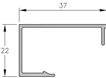
1110051 - Contravidrio recto 37 mm para clip Largo Std.: 6030 mm peso: 0,27 Kg/m
