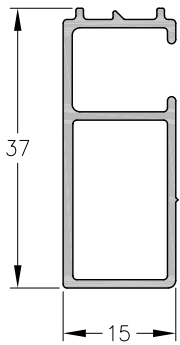
1020718 - Premarco 36 mm Largo Std.: 6150 mm peso: 0,33 Kg/m
