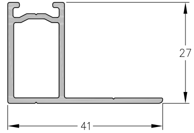
1110069 - Guía fija móvil Peso: 0,42 Kg/m Largo Std.: 6150 mm
