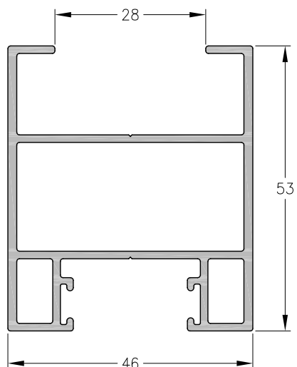
1110716 - Parante lat hoja 90° DVH 28 mm Largo Std.: 6150 mm peso: 1,04 Kg/m
