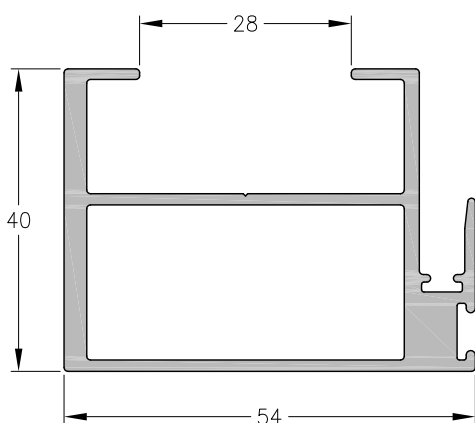
1110717 - Parante cent hoja 90° DVH 28 mm Largo Std.: 6150 mm peso: 1,16 Kg/m
