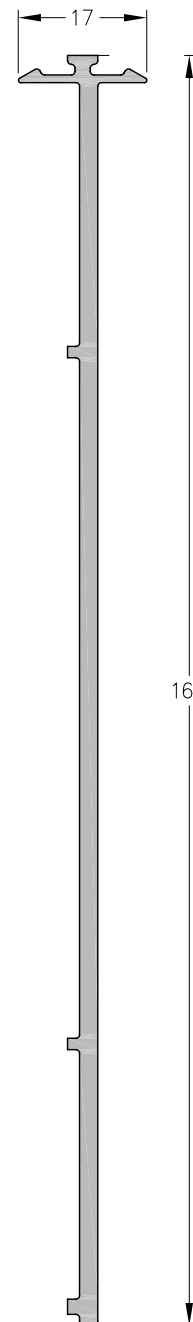
1110701 - Acople 3 guías Peso: 1,16 Kg/m Largo Std.: 6150 mm
