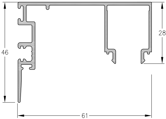
1110068 - Cierre parante F/M Peso: 0,71 Kg/m Largo Std.: 6030 mm
