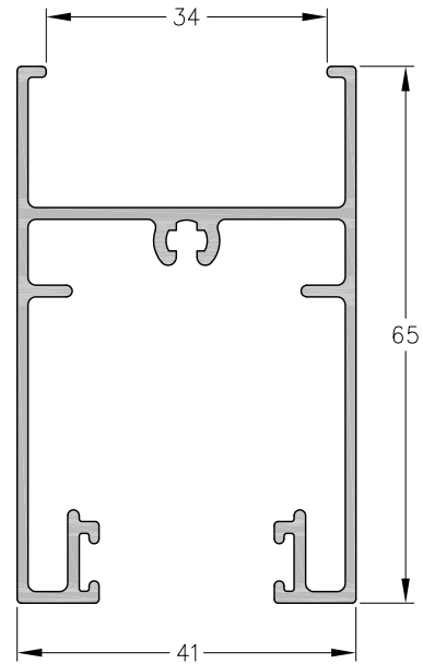
1110868 - Zócalo y cabezal hoja corte 90° DVH Peso: 0,89 Kg/m Largo Std.: 6030 mm
