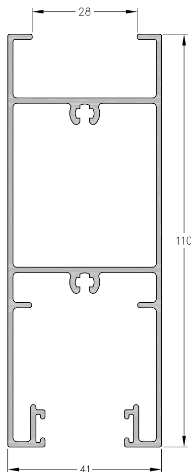
1110728 - Zócalo alto hoja 90° DVH 28 mm Largo Std.: 6030 mm peso: 1,49 Kg/m
