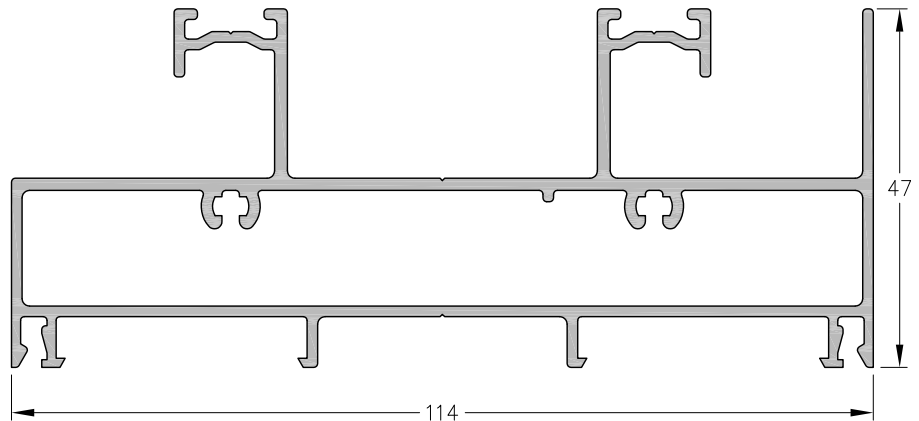
1110864 - Umbral / dintel marco corrediza 2 guías Peso: 1,79 Kg/m Largo Std.: 6150 mm
