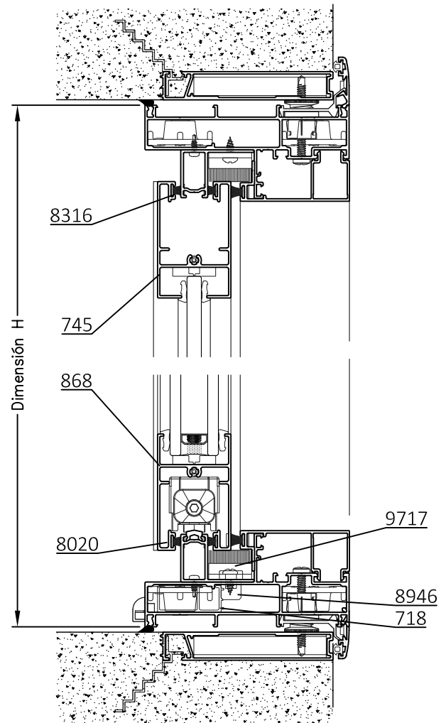
C-C Corte Vertical
