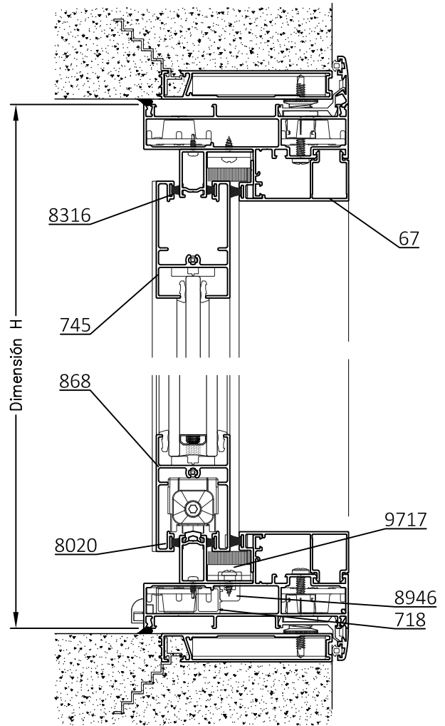
C-C Corte Vertical
