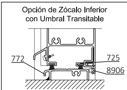
A-A Corte Horizontal
