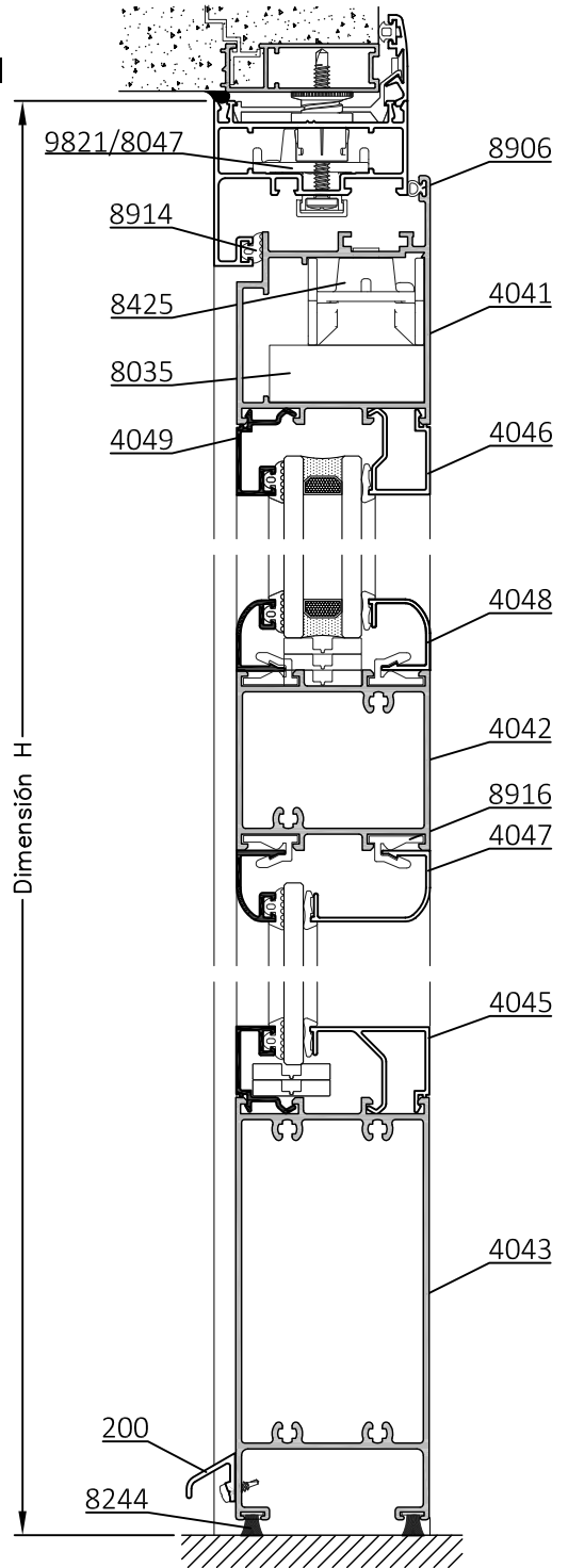
B-B Corte Vertical (Con Travesaño)
