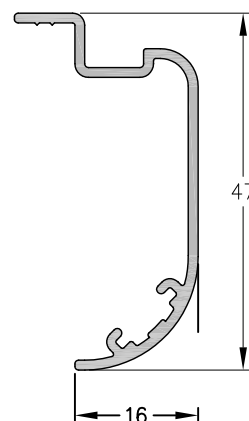
1020641 - Contramarco peso: 0,32 Kg/m
