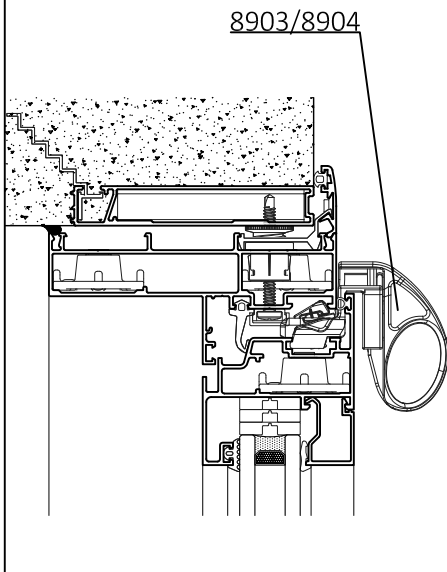
Corte C
