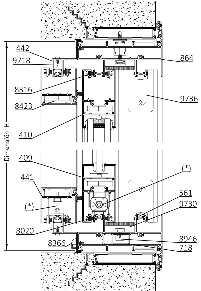
B-B Corte Vertical
