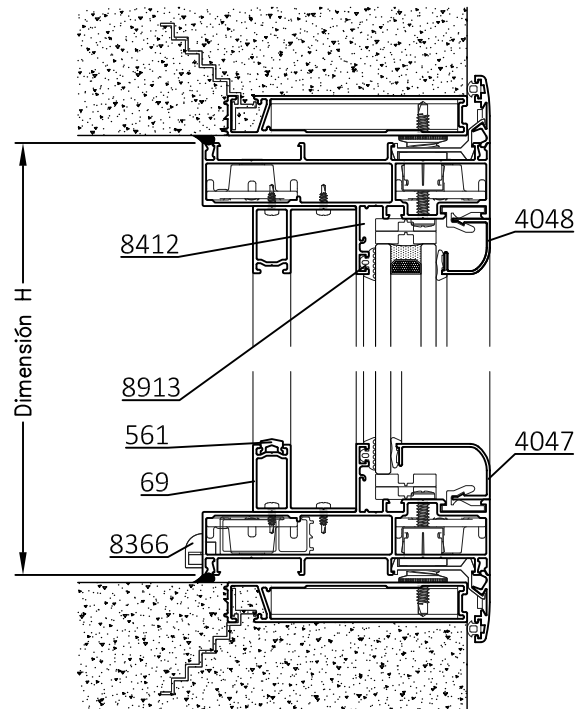
B-B Corte Vertical
