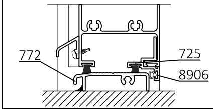
Opción de Zócalo Inferior con Umbral Transitable
