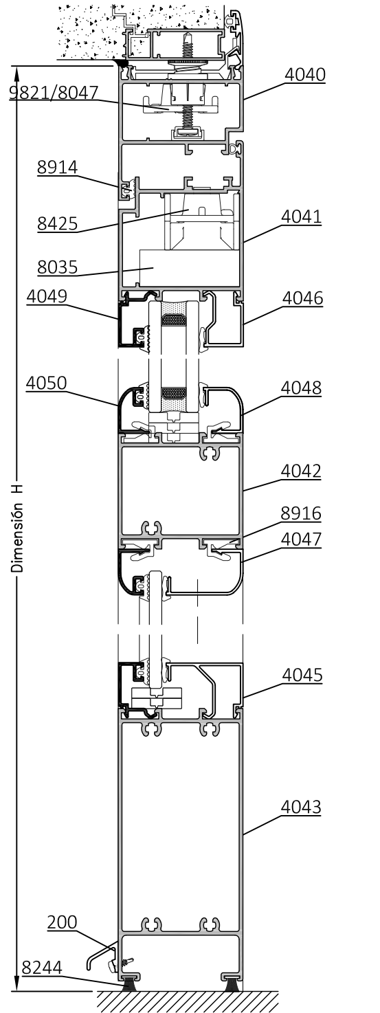
B-B Corte Vertical (Con Travesaño)
