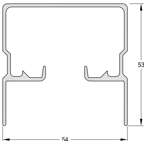
1090941 - Cabezal Peso: 0,82 Kg/m. Largo Std.: 6.030 mm.
