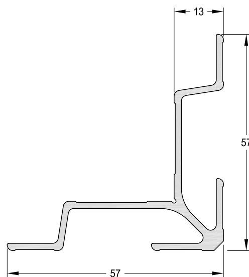
1090063 - Escuadra Universal Pesada Peso: 0,74 Kg/m. Largo Std.: 6.030 mm.
