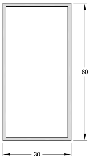
1090813 - Tubo 60 x 30 mm. Peso: 0,68 Kg/m. Largo Std.: 6.030 mm.
