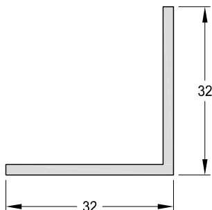
1090756 - Perfil Angulo Peso: 0,34 Kg/m. Largo Std.: 6.030 mm.
