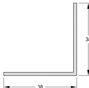
1090757 - Perfil Angulo Peso: 0,34 Kg/m. Largo Std.: 6.030 mm.
