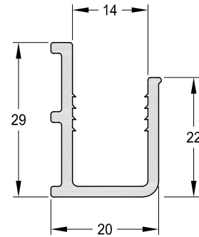
1090031 - Porta Blisan Inferior Peso: 0,38 Kg/m. Largo Std.: 6.030 mm.
