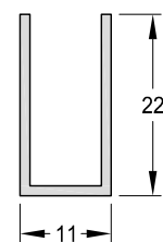
1090466 - "U" 11,1 x 22 mm Peso: 0,17 Kg/m. Largo Std.: 6.030 mm.
