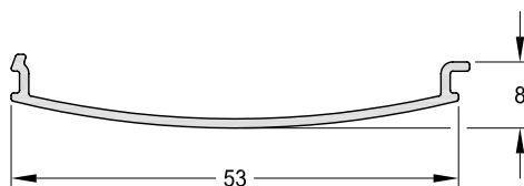
1090029 - Tapa Inferior Pasamanos Curvo Peso: 0,20 Kg/m. Largo Std.: 6.030 mm.
