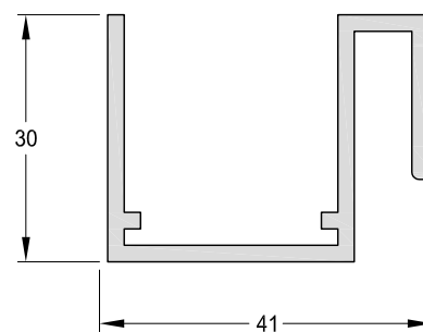
3079 - Perfil Bandeja "S" Peso: 0,64 Kg/m. Largo Std.: 6.030 mm.
