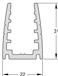
1090201 - Marco Peso: 0,52 Kg/m. Largo Std.: 6.030 mm.
