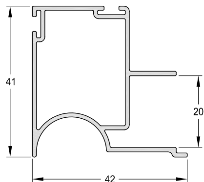
1090159 - Parante de 18 mm. Peso: 0,54 Kg/m. Largo Std.: 5.200 mm.
