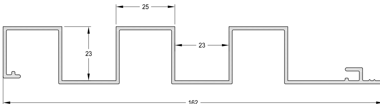
3112 - Revestimiento 25 - 23 - 23 Peso: 1,20 Kg/m. Largo Std.: 6.200 mm.
