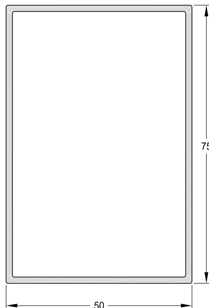
1090464 - Tubo 75 x 50 mm. Peso: 1,12 Kg/m. Largo Std.: 6.030 mm.
