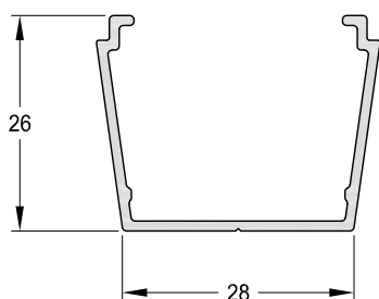
1090631 - CLIP Parasol 25 mm Largo Std.: 6030 mm peso: 0,279 Kg/m
