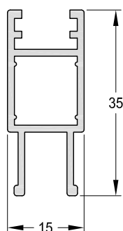
1090944 - Hoja Peso: 0,35 Kg/m. Largo Std.: 6.030 mm.
