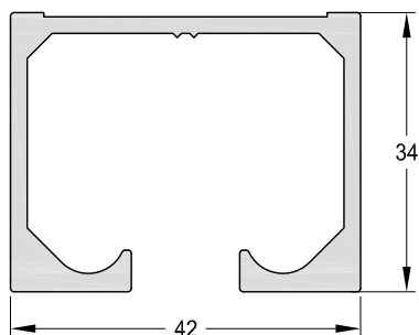
3082 - Riel Corredizo Sup. R164 Peso: 0,86 Kg/m. Largo Std.: 6.030 mm.
