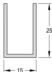
1090650 - "U" de Blindex Peso: 0,25 Kg/m. Largo Std.: 6.030 mm.
