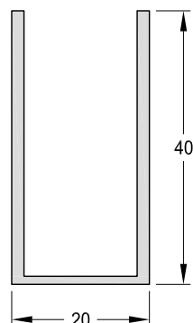
3043 - "U" 40 x 20 mm Peso: 0,46 Kg/m. Largo Std.: 6.030 mm.
