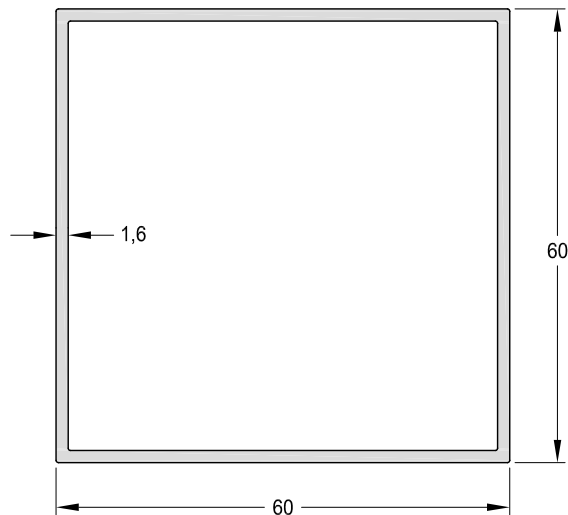
1090459 - Tubo 60 x 60 mm. Peso: 1,01 Kg/m. Largo Std.: 6.030 mm.
