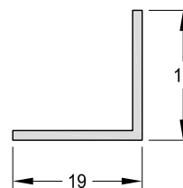
1090753 - Perfil Angulo Peso: 0,14 Kg/m. Largo Std.: 6.030 mm.
