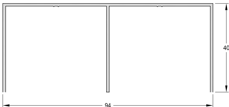
1090160 - Guía Superior Peso: 0,68 Kg/m. Largo Std.: 6.030 mm.
