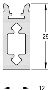
1090202 - Porta Hoja Peso: 0,57 Kg/m. Largo Std.: 6.030 mm.
