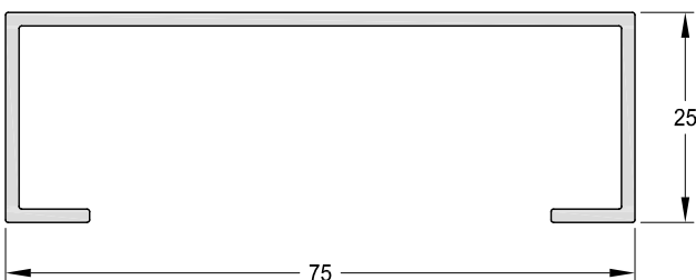
1090118 - Canal Liso 75 x 25 mm. Peso: 0,60 Kg/m. Largo Std.: 6.030 mm.
