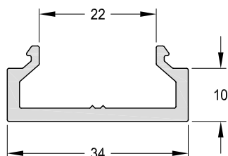
1090111 - Suplemento Zócalo Peso: 0,39 Kg/m. Largo Std.: 6.030 mm.
