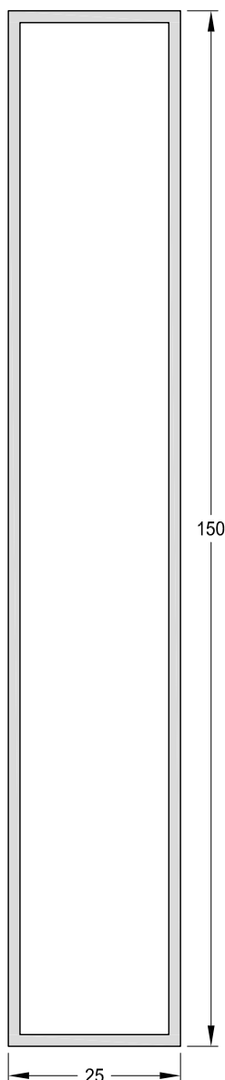
1090472 - Tubo 150 x 25 mm. Peso: 1,58 Kg/m. Largo Std.: 6.030 mm.
