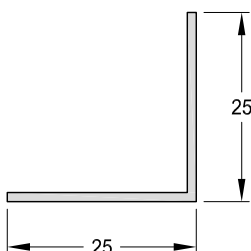
1090755 - Perfil Angulo Peso: 0,16 Kg/m. Largo Std.: 6.030 mm.
