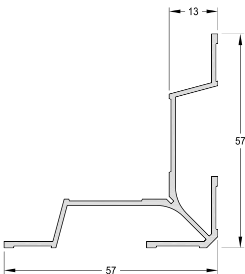
1090055 - Escuadra Universal Intermedia Peso: 0,56 Kg/m. Largo Std.: 6.030 mm.
