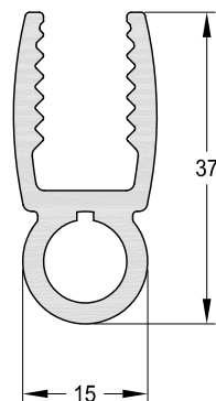
1090203 - Hoja Peso: 0,64 Kg/m. Largo Std.: 6.030 mm.
