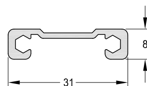
1090946 - Barra Toallera Peso: 0,24 Kg/m. Largo Std.: 6.030 mm.
