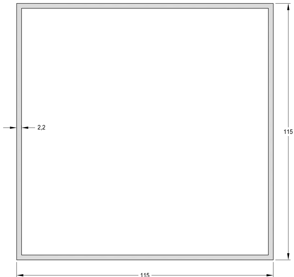
1090700 - Tubo 115 x 115 mm. Peso: 2,68 Kg/m. Largo Std.: 6.150 mm.
