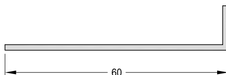
1090124 - Perfil Angulo Peso: 0,64 Kg/m. Largo Std.: 6.030 mm.
