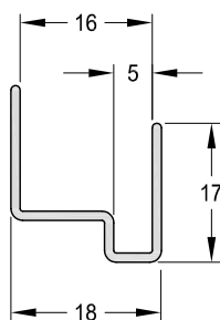
1090156 - Cantonera de 15 mm. Peso: 0,16 Kg/m. Largo Std.: 6.030 mm.
