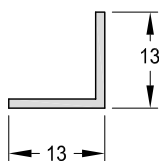
1090751 - Perfil Angulo Peso: 0,08 Kg/m. Largo Std.: 6.030 mm.
