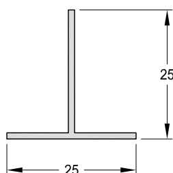
1090830 - Perfil T Peso: 0,16 Kg/m. Largo Std.: 6.030 mm.
