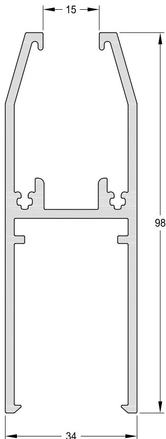
1090110 - Zócalo Peso: 1,66 Kg/m. Largo Std.: 6.030 mm.
