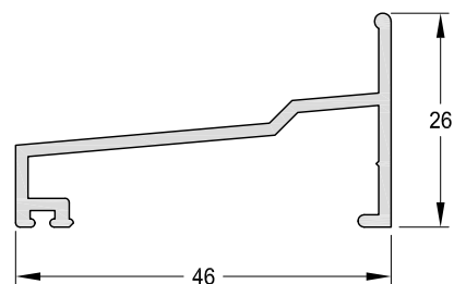
1090942 - Umbral Peso: 0,37 Kg/m. Largo Std.: 6.030 mm.
