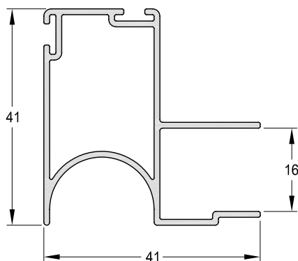
1090155 - Parante de 15 mm. Peso: 0,53 Kg/m. Largo Std.: 5.200 mm.
