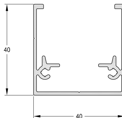
1090630 - Base Parasol 25 mm Largo Std.: 6030 mm peso: 0,642 Kg/m
