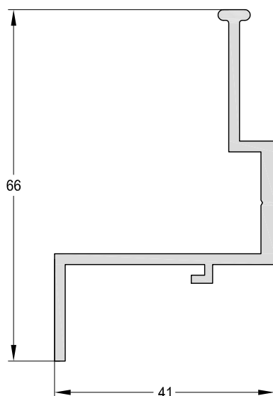
3078 - Perfil Bandeja "Z" Peso: 0,67 Kg/m. Largo Std.: 6.030 mm.
