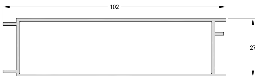
3084 - Revestimiento Tubular E27 mm. Peso: 0,97 Kg/m. Largo Std.: 6.030 mm.
