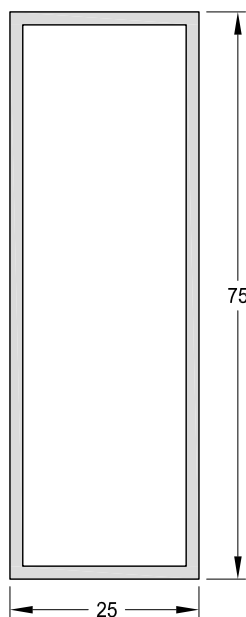
1090457 - Tubo 75 x 25 mm. Peso: 0,90 Kg/m. Largo Std.: 6.030 mm.
