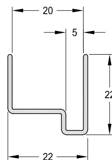
1090158 - Cantonera de 18 mm. Peso: 0,20 Kg/m. Largo Std.: 6.030 mm.
