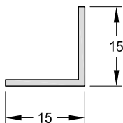
1090752 - Perfil Angulo Peso: 0,10 Kg/m. Largo Std.: 6.030 mm.
