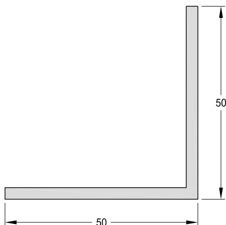
1090759 - Perfil Angulo Peso: 0,79 Kg/m. Largo Std.: 6.030 mm.
