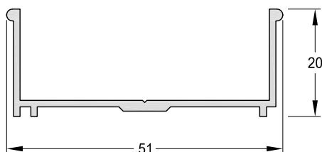
1090943 - Jamba Peso: 0,32 Kg/m. Largo Std.: 6.030 mm.
