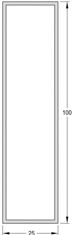
1090461 - Tubo 100 x 25 mm. Peso: 0,99 Kg/m. Largo Std.: 6.030 mm.
