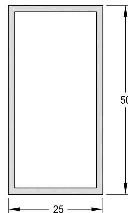
1090809 - Tubo 50 x 25 mm. Peso: 0,55 Kg/m. Largo Std.: 6.030 mm.
