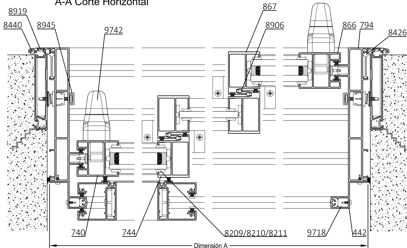
A-A Corte Horizontal
