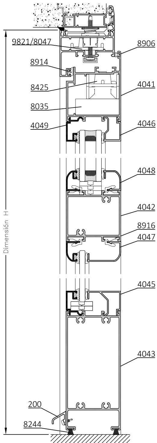
B-B Corte Vertical (Con Travesaño)
