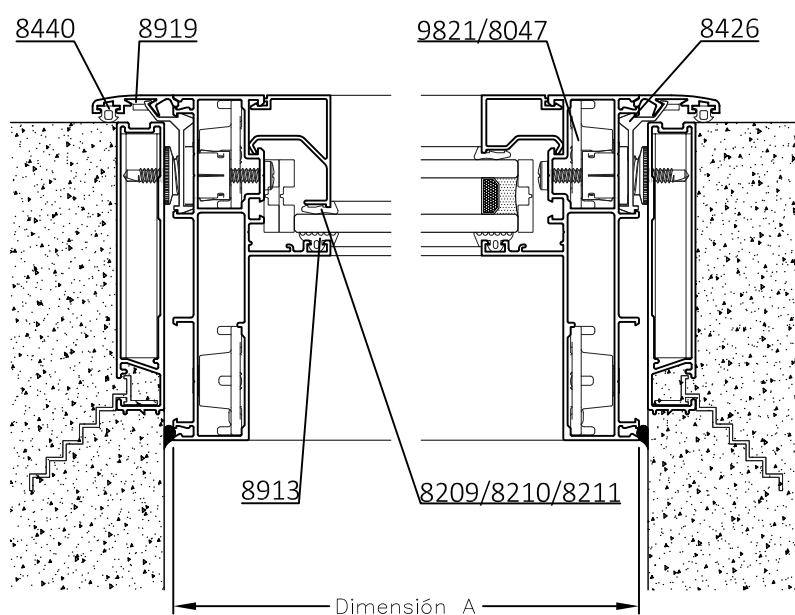
A-A Corte Horizontal
