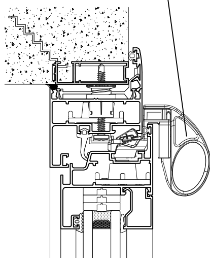
Corte C
