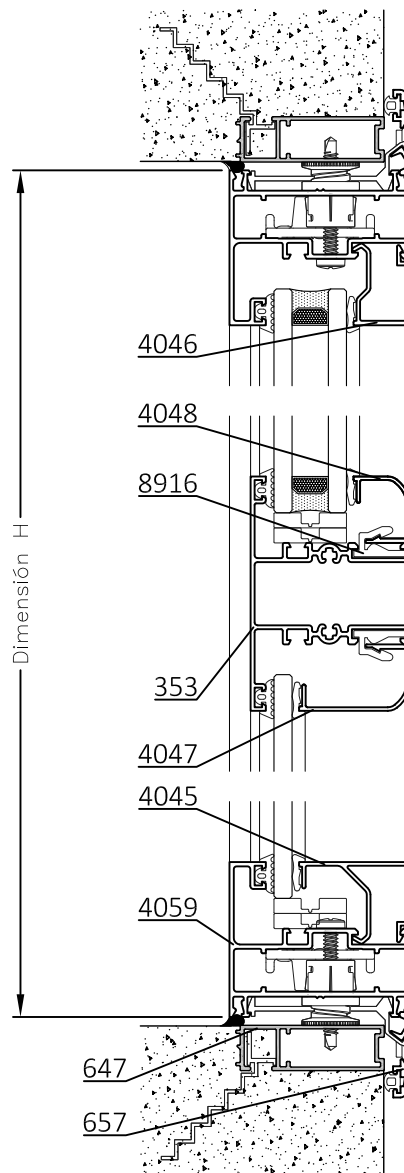
B-B Corte Vertical
