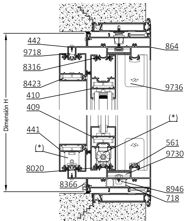
B-B Corte Vertical
