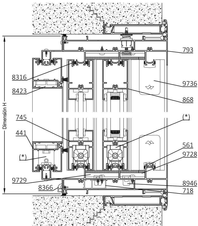
B-B Corte Vertical
