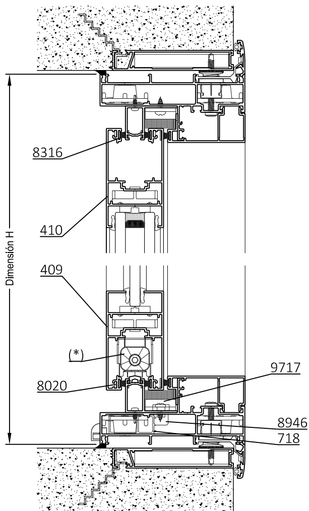
B-B Corte Vertical
