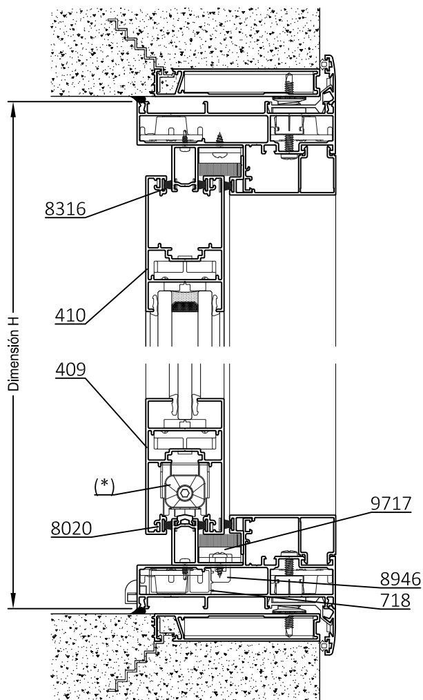
C-C Corte Vertical
