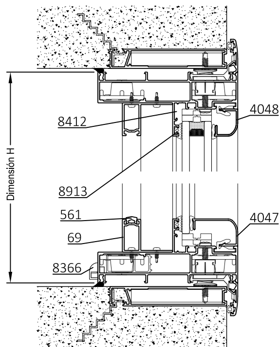
C-C Corte Vertical
