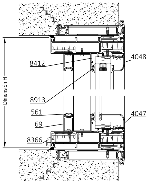
A-A Corte Horizontal
