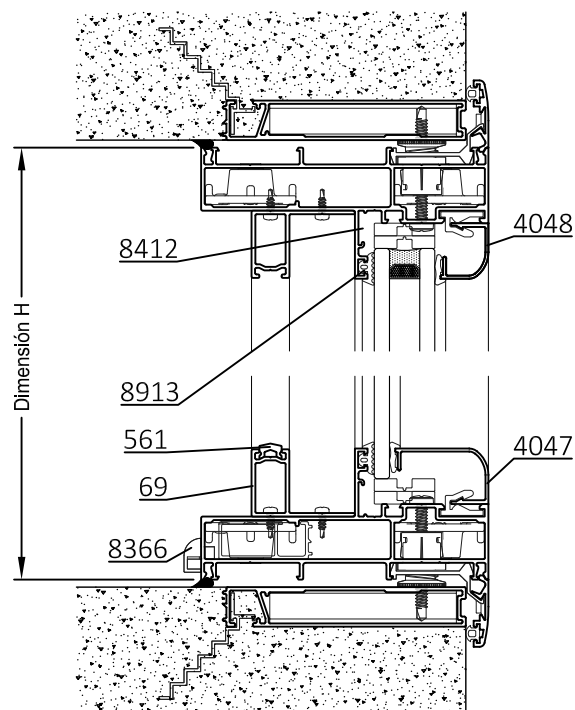
B-B Corte Vertical
