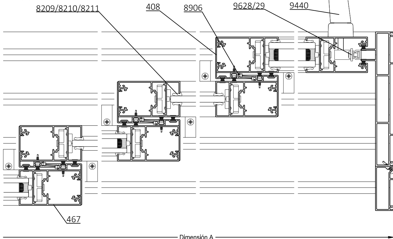
A-A Corte Horizontal
