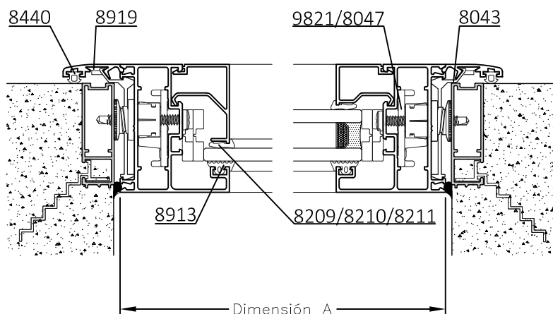
A-A Corte Horizontal
