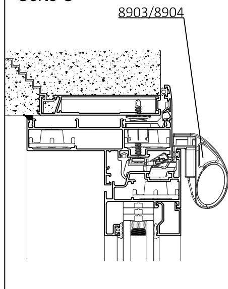
Corte C
